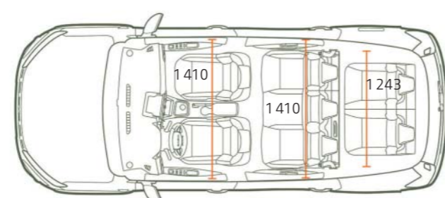
OBERANSICHT 7-PLÄTZER
