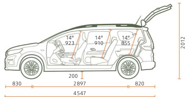
SEITENANSICHT 7-PLÄTZER
