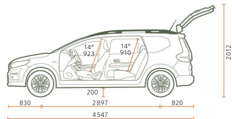
SEITENANSICHT 5-PLÄTZER
