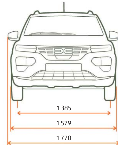
FRONTANSICHT
